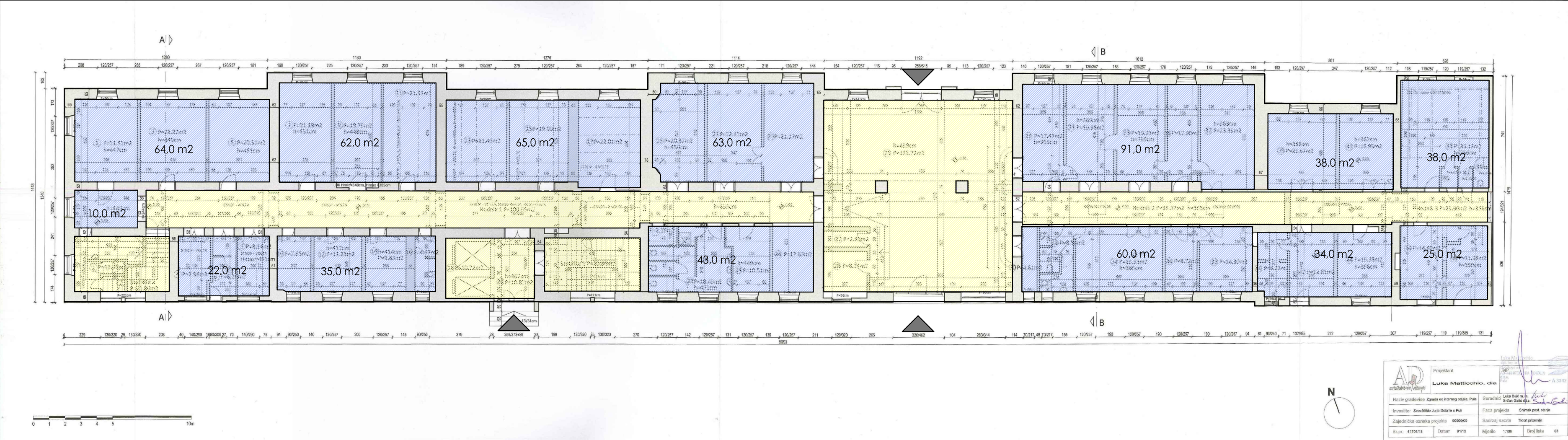
TLOCRT PRIZEMLJA
